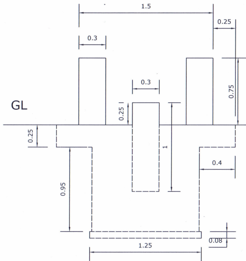
ELEVATION
