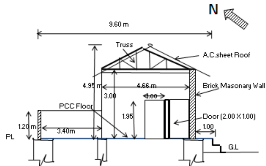
SECTION -- AB
