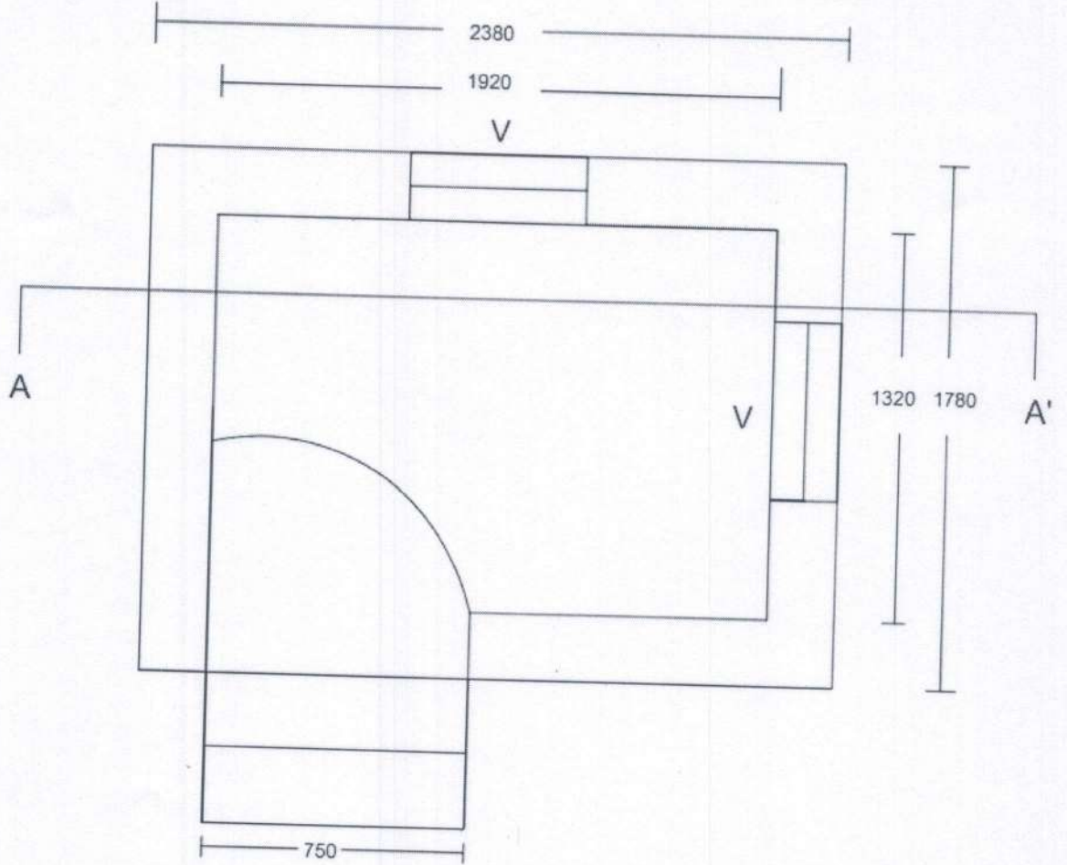
Toilet Plan
