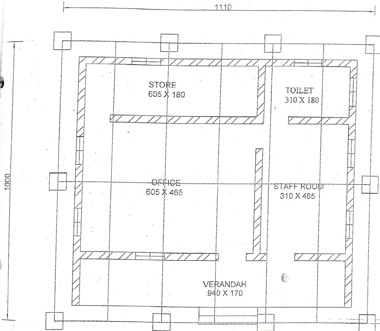
SITE OFFICE MANKARA -PLAN
